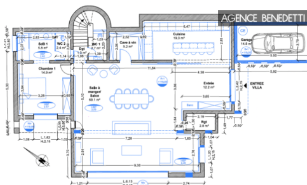
PLAN R-1 PROJET 1/100
