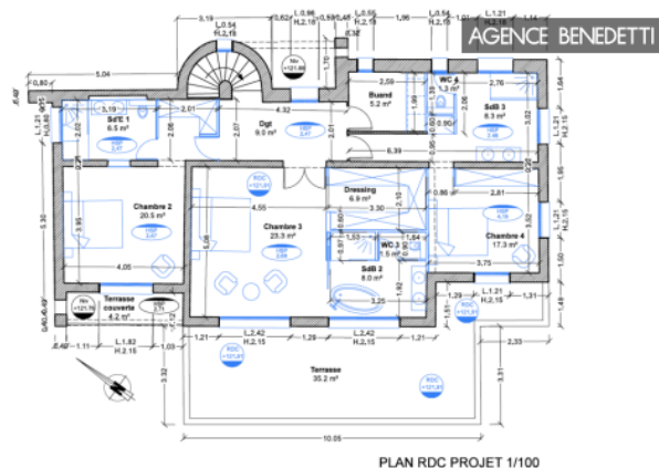
PLAN RDC PROJET 1/100
